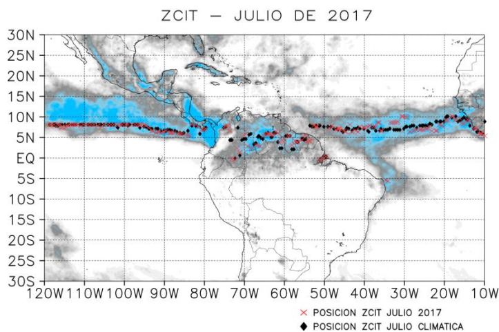
Fig. N°8. Posición mensual de la ZCIT en el Pacífico ecuatorial. Fuente: TRMM-3B42-RT (satélite) – SPC/SENAMHI.
