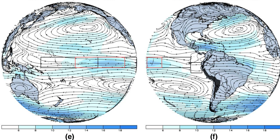
Fig. N°3. Flujo total (líneas) y zonal (colores) del viento en el Pacífico en tropósfera baja. Fuente: CPC/NCEP-Elaborado por SPC/SENAMHI.
