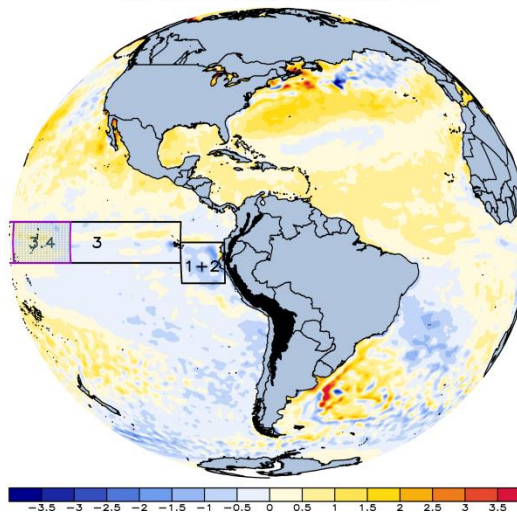
Fig. N°1. TSM (panel superior)/ATSM (panel inferior). Fuente: AVHRR-NOAA – Elaborado por SPC/SENAMHI.
