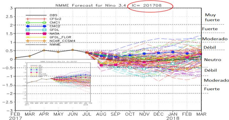
Fig. N°15. Pronóstico ENSO en el Pacífico ecuatorial central. Fuente: IRI / CPC.
