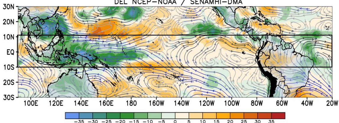
Fig. N°7. Anomalías espaciales de ROL en w/m2. Valores negativos (positivos) de ROL (coloración verde-azul/ amarillo - rojo) reflejan zonas con mayor (menor) nubosidad a lo normal, donde zonas con valores más bajos (altos) corresponden a regiones que presentaron precipitaciones por encima (debajo) de lo normal. Flujo anómalo del viento en 925 hPa (-700 msnm). Fuente: CPC/NCEP – Elaborado por SPC/SENAMHI.
