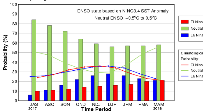
Salida Consensuada IRI/CPC Inicios de Agosto 2017. Early-Aug CPC/IRI Official Probabilistic ENSO Forecast
