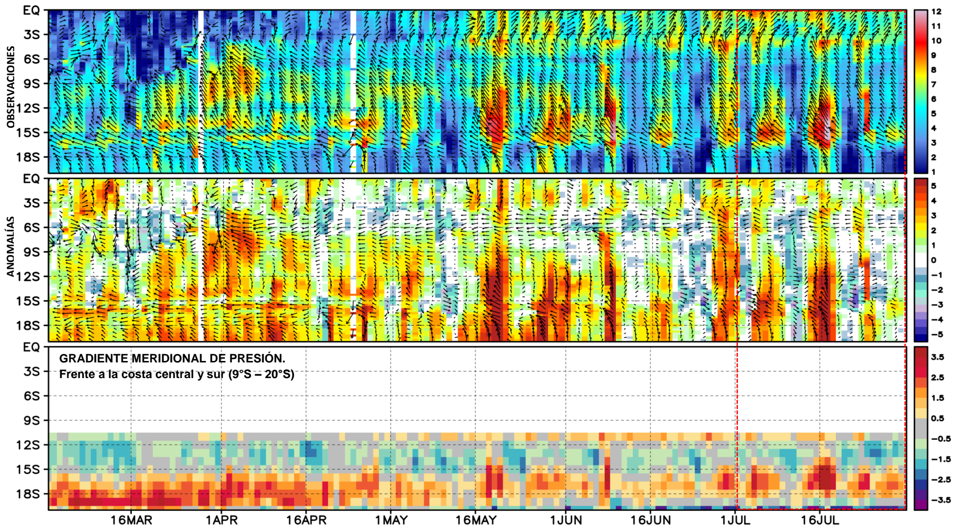
Fig. N°14. Evolución espacio – temporal del viento costero ( m*s^{-1} , 10m de la superficie oceánica) y el gradiente meridional de presión (AGP), ambos hasta ~100 Km fuera de la costa peruana. Fuente: NESDIS-NOAA/SENAMHI DMA-SPC.
