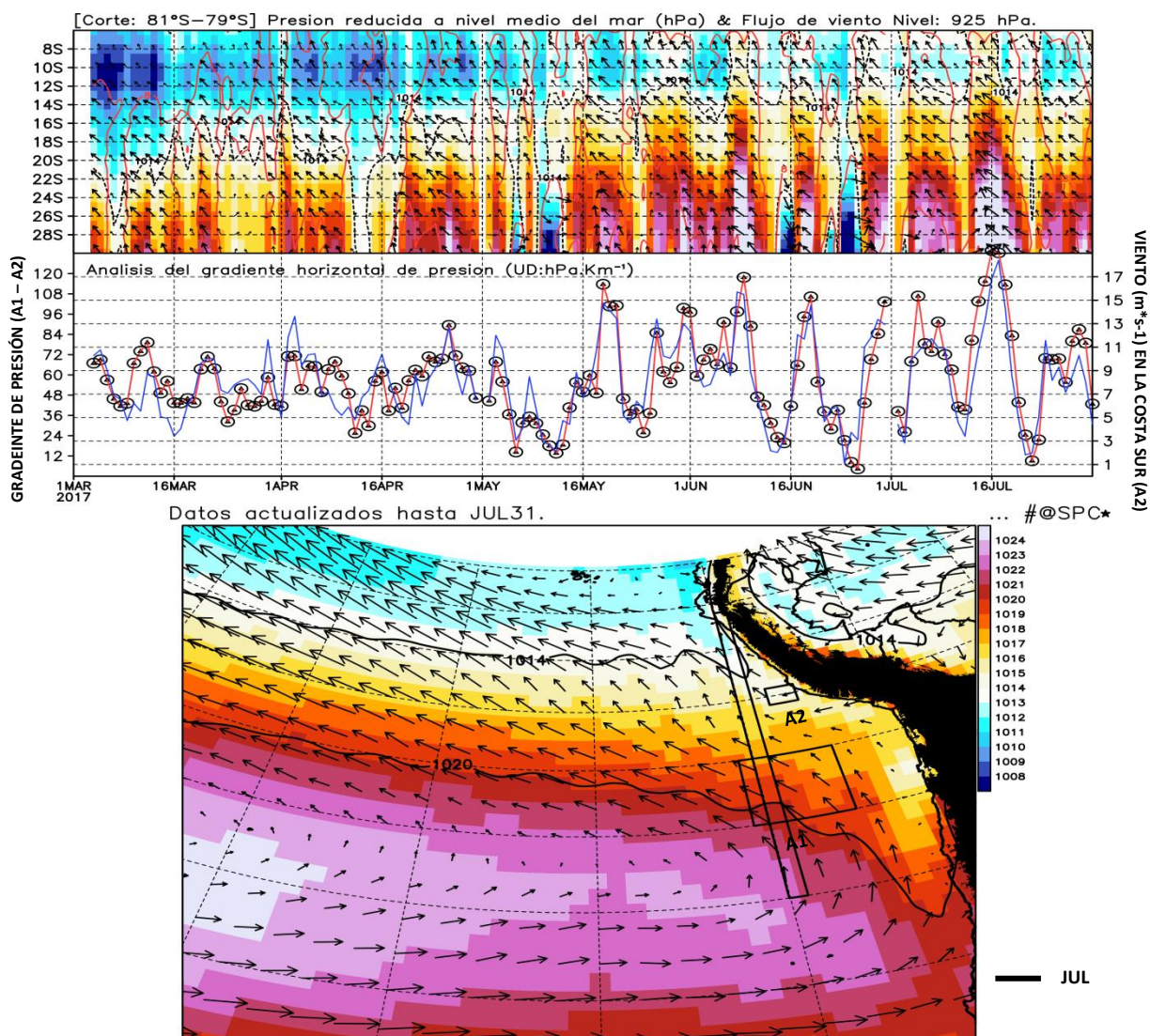
Fig. N°13. Evolución espacio – temporal de la intensidad diaria del APSE y el gradiente horizontal de presión frente a la costa oeste de Sudamérica (panel superior). Evolución mensual de las isóbaras de 1010, 1014 y 1020 hPa, y viento en 850 hPa (panel inferior). Fuente: SENAMHI/DMA-SPC.
