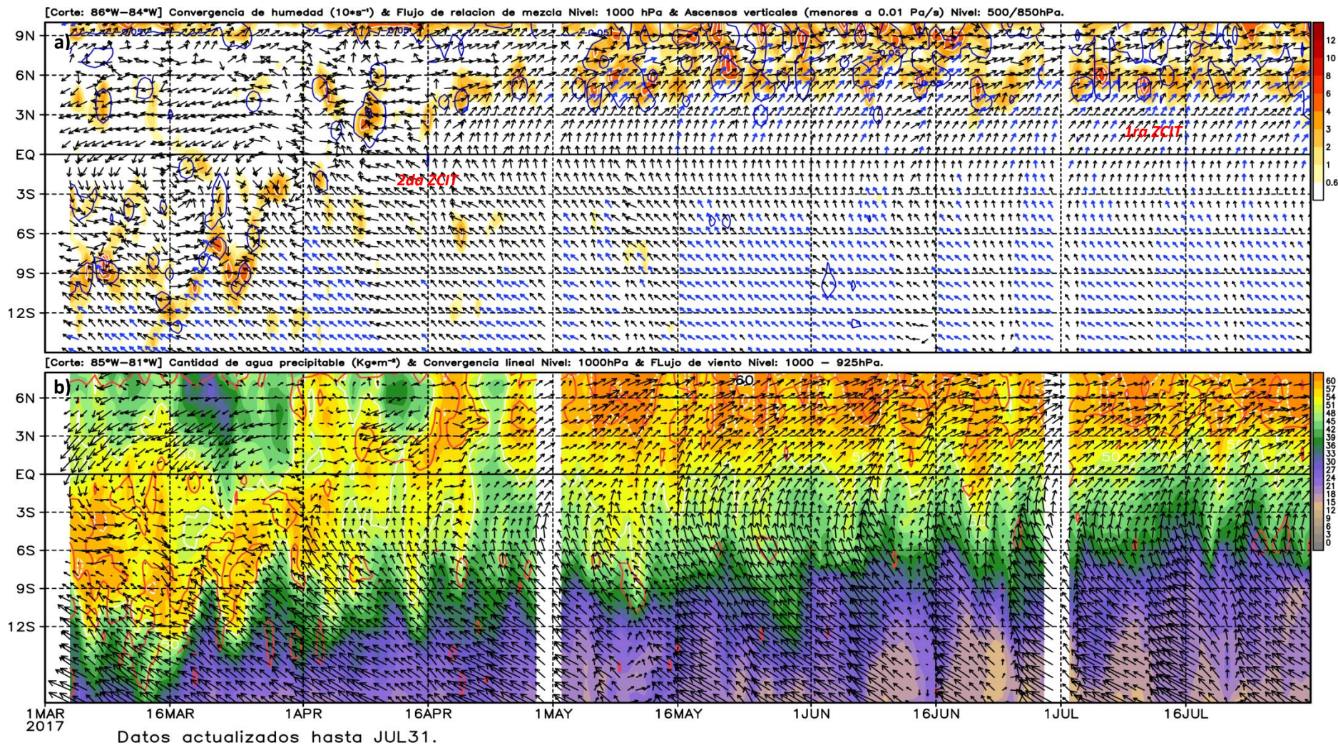
Fig. N°12. Evolución latitudinal de patrones atmosféricos relevantes frente a la costa norte. Fuente: SENAMHI/DMA-SPC.
