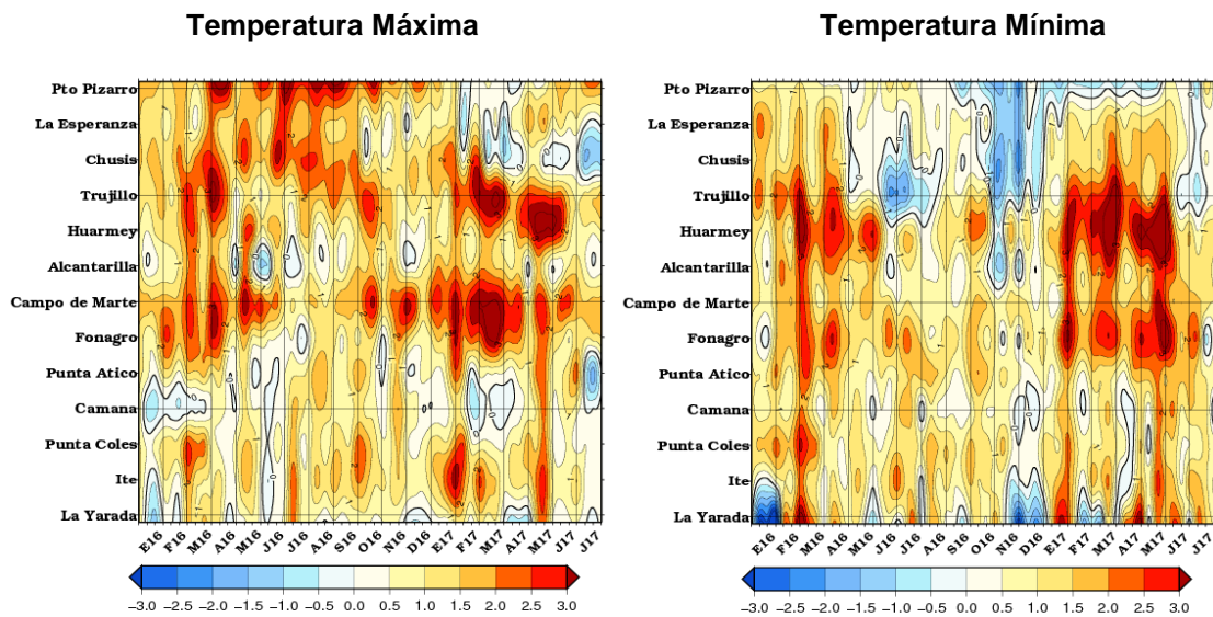
Fig. N°11. Evolución decadiaria de las temperaturas extremas del aire. Fuente: SENAMHI/SPC.
